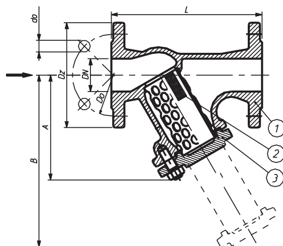
Rys. 1 Budowa i wymiary filtra
